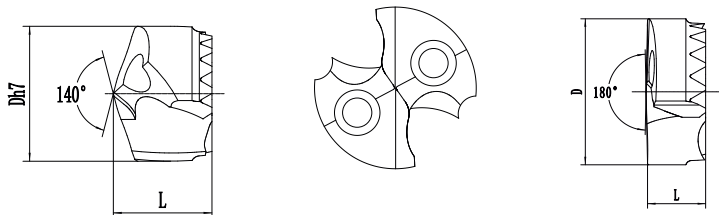
剑齿钻头型号及尺寸
