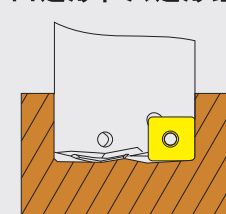
四边形和六边形组合刀片浅孔钻
