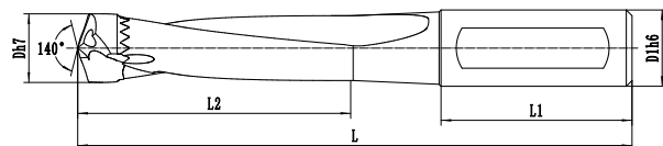
剑齿钻刀杆型号及尺寸
