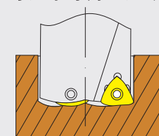
等边不等角六边形刀片浅孔钻
